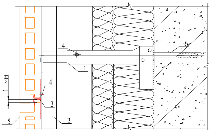
Горизонтальный стык плит облицовки (крепление на кляммерах)
